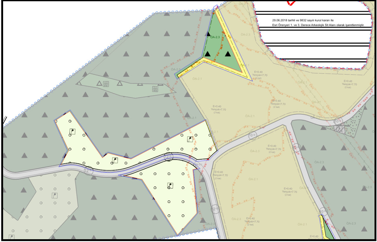
Şekil 2. Teklif 1/1000 ölçekli Uygulama İmar Planı
