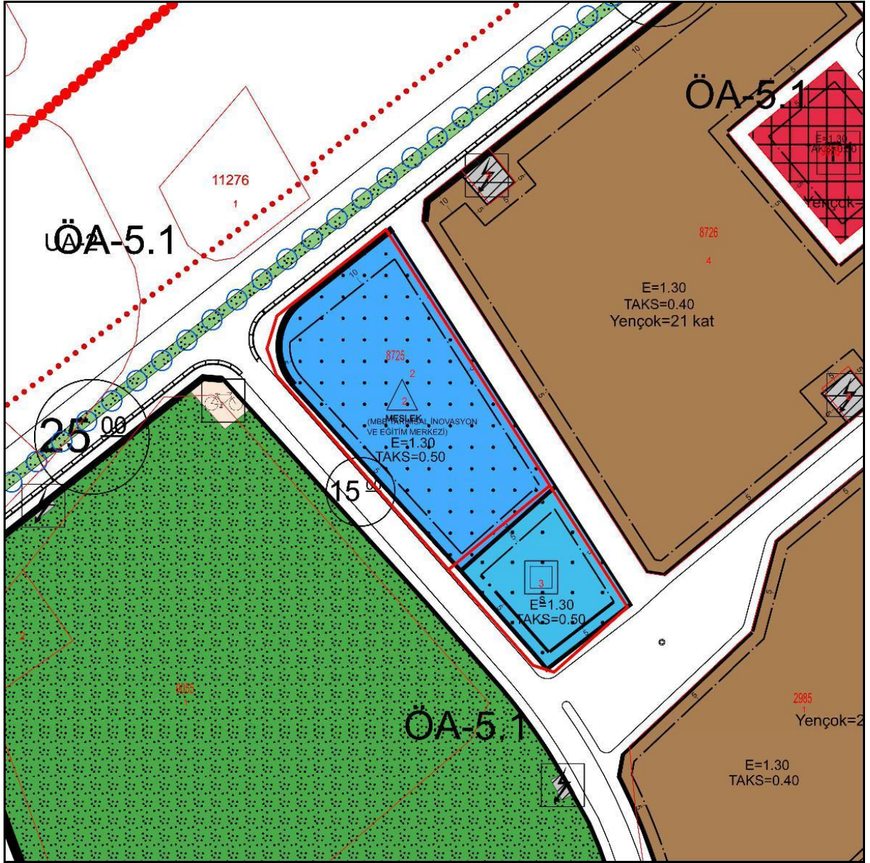
Şekil 3. Yürürlükteki 1/1000 Ölçekli Uygulama İmar Planı
