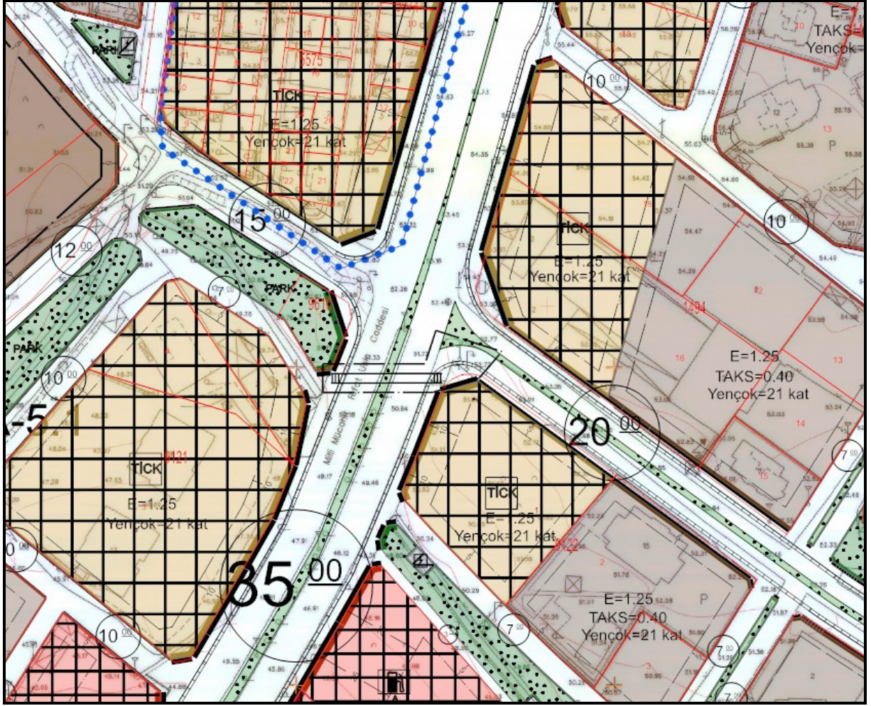
Şekil 3. 1/1000 Ölçekli Uygulama İmar Planı Değişikliği Teklifi
