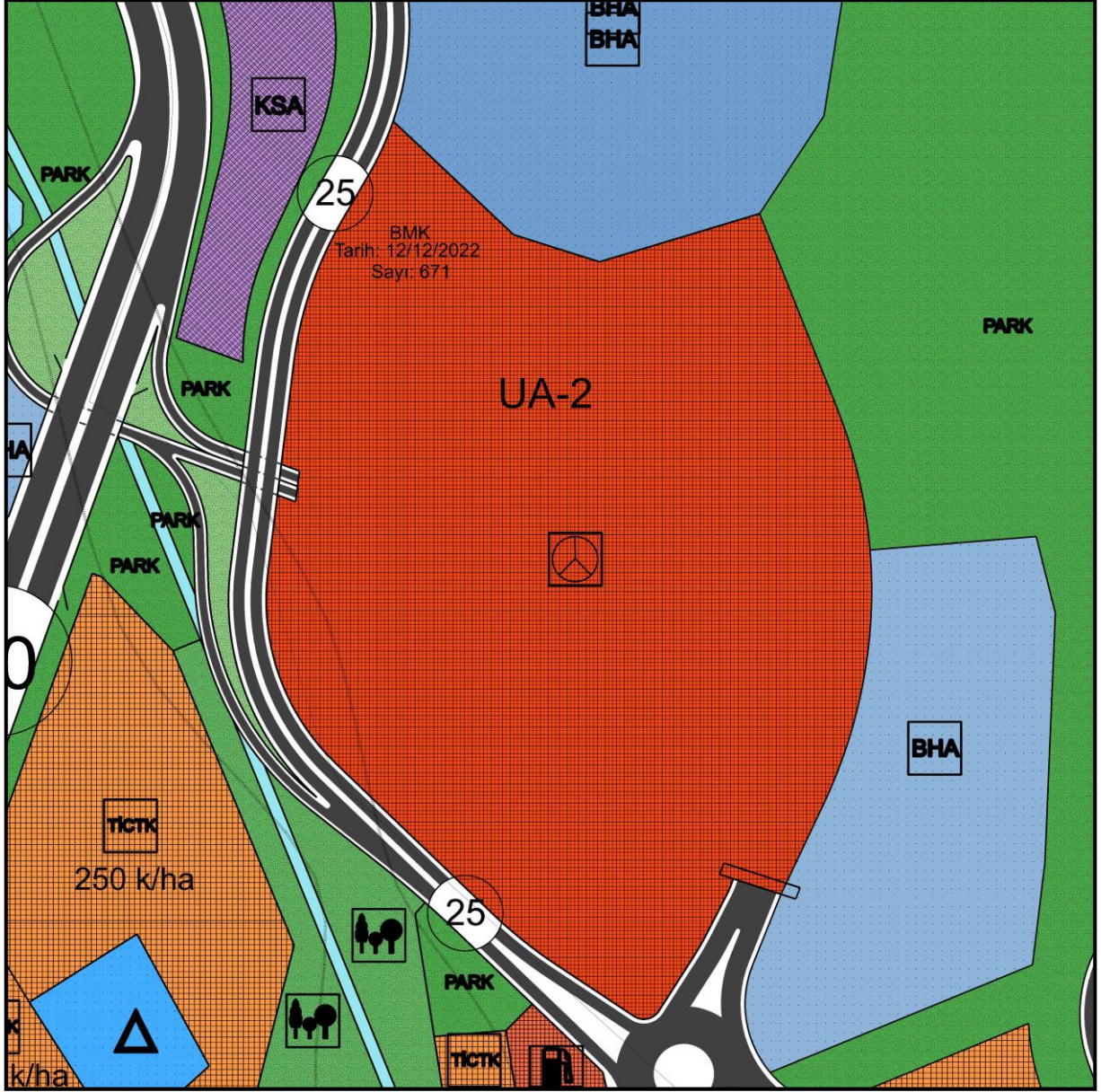
Şekil 2. Yürürlükte bulunan 1/5000 ölçekli Nazım İmar Planı
